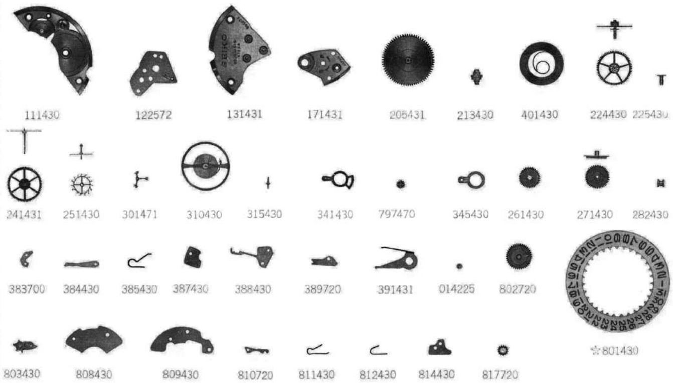
キャリバー No. 5722B
