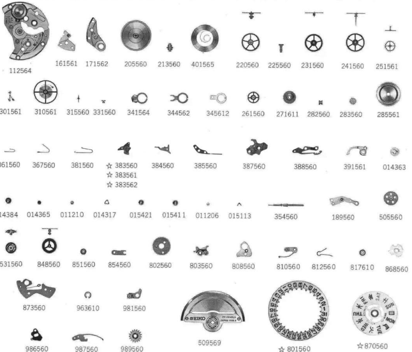
キャリバーNo.5646A
